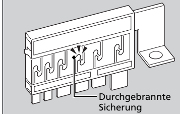
Kombi-Sicherung
