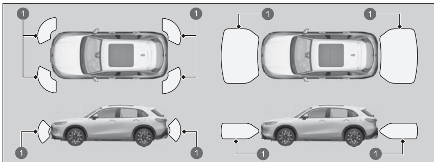
1 Sonar-Reichweite
