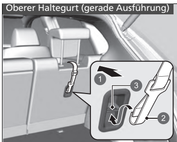
1 Fahrtrichtung 2 Haltegurt 3 Verankerung
