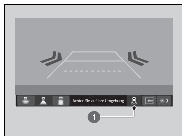
1 Symbol für den Ausparkassistenten
