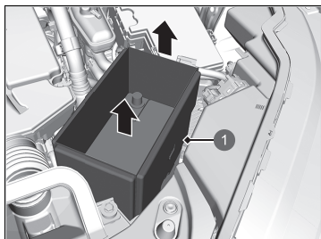
1 Batterieabdeckung
