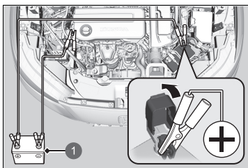
1 Hilfsbatterie
