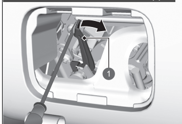
1 Hebel
