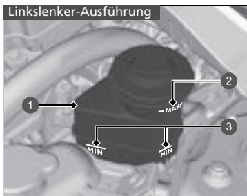
Linkslenker-Ausführung
