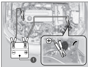
1 Hilfsbatterie
