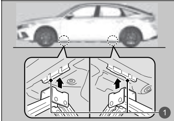
1 Hebepunkte
