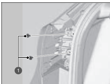
1 Schrauben
