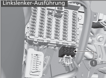
1 Sicherungskasten B
